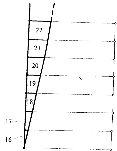
แผนที่ส่วนขยายแนวเขตที่ดินที่ต้องเวนคืน มาตราส่วน 1 : 500
